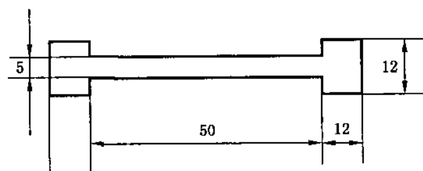
图 3 哑铃试样
