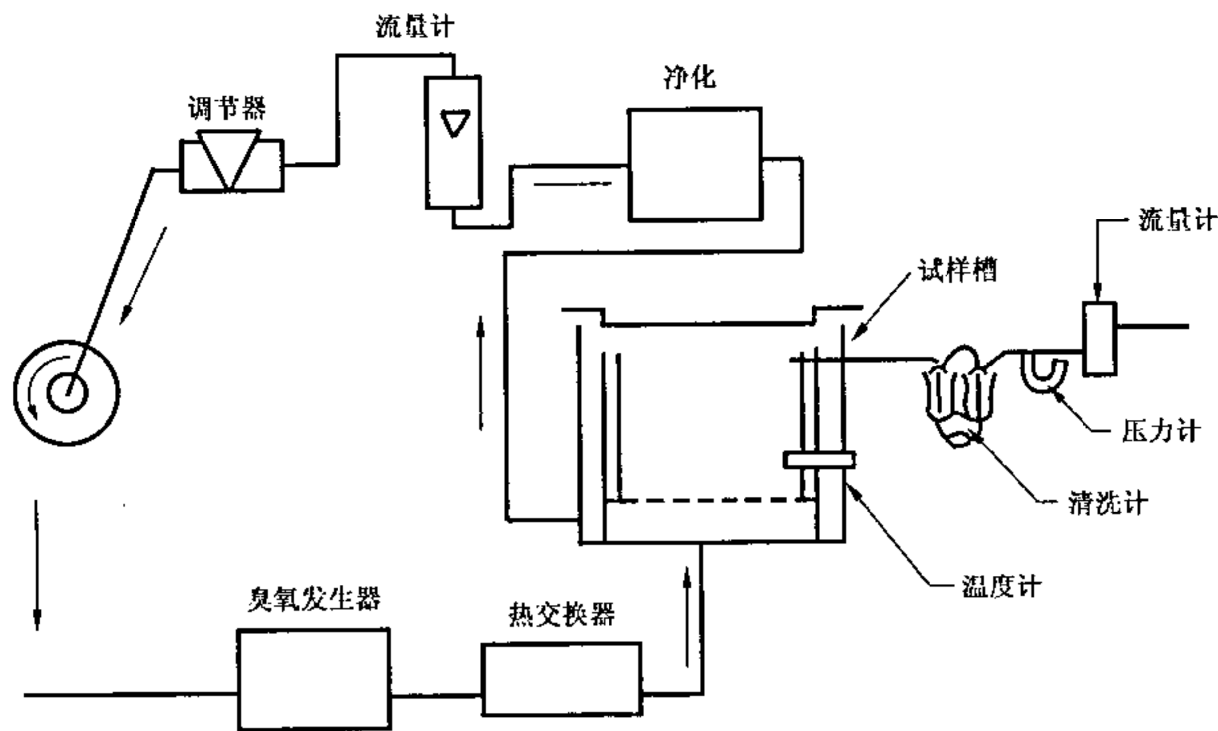
图 1 试验装置示意图
