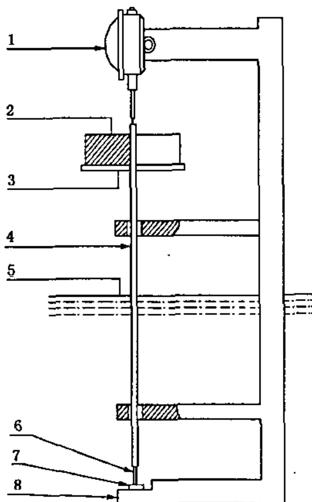
1—千分表;2—砝码;3—载荷盘;4—负载杆; 5—液面;6—压针;7—试样;8—试样支架
