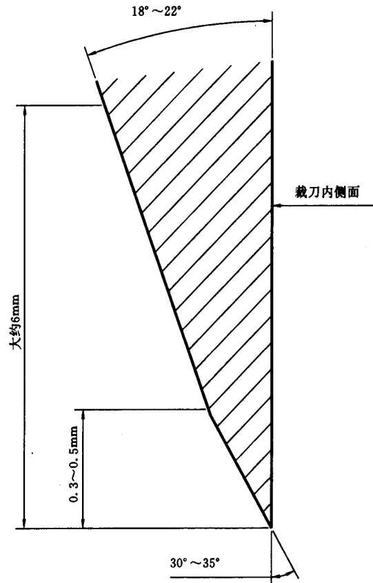
图 1 裁刀的刃口
