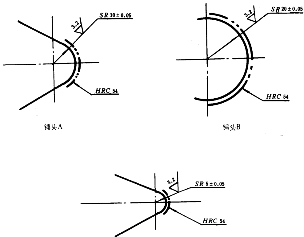
锤头C
