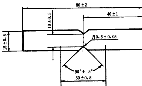
图 5 E 型试样
