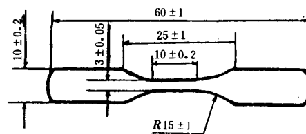
图 3 C 型试样
