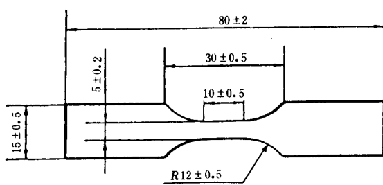
图 2 B 型试样
