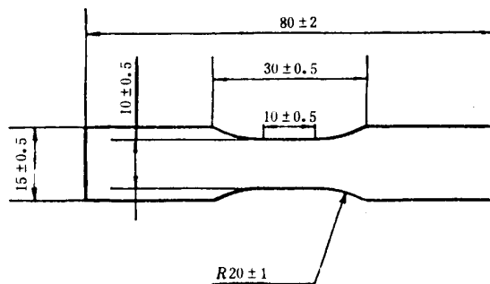
图 1 A 型试样
