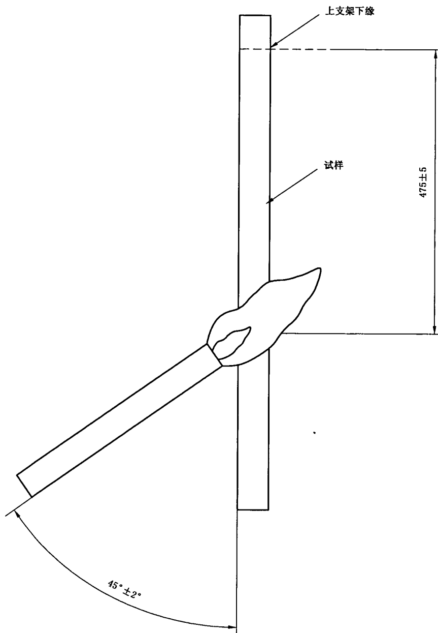
图 2 对试样供火
