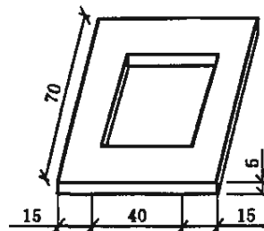
图1 粘接强度试件成型模框
